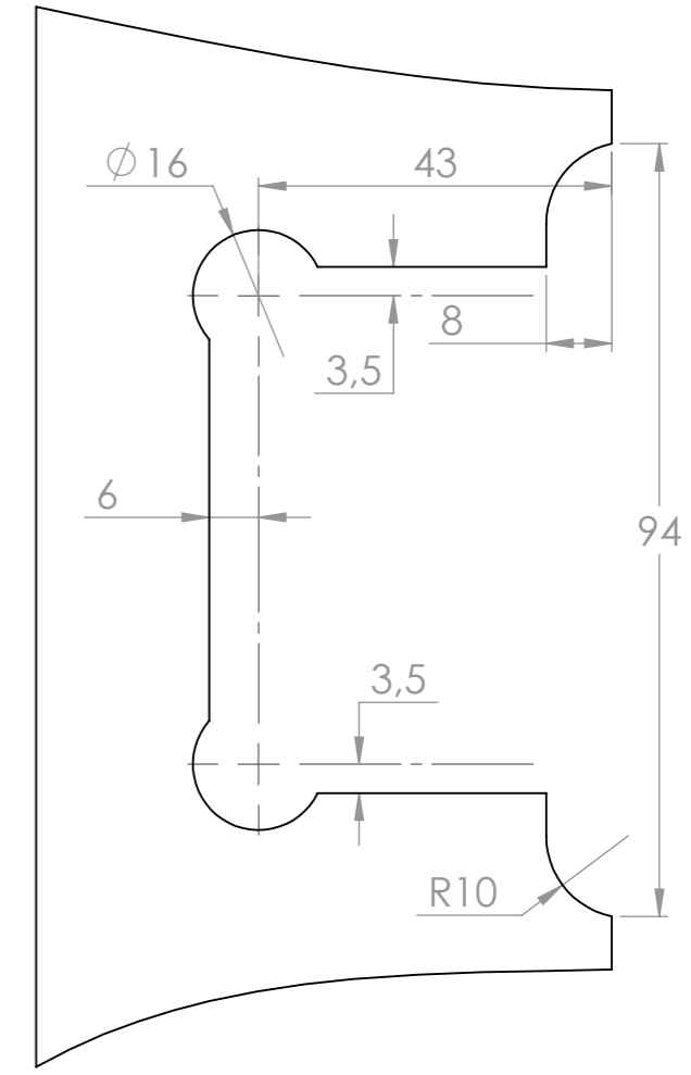
Zonder afdichtingsprofiel
