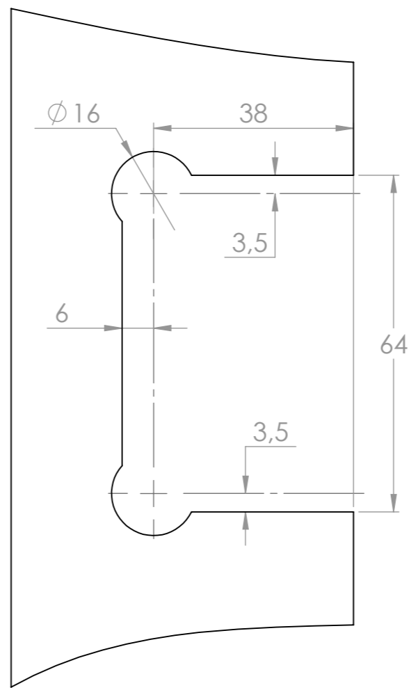
Met afdichtingsprofiel
