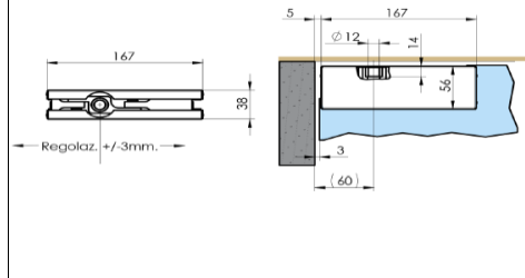
Uitsparing bovenkant 100E20 - Encoche en haut 100E20 Notch at the top 100E20
