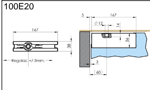
Uitsparing bovenkant 100E20 - Encoche en haut 100E20 Notch at the top 100E20
