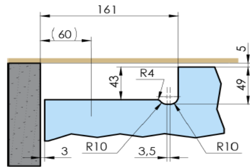
Uitsparing bovenkant 100E20 - Encoche en haut 100E20 Notch at the top 100E20
