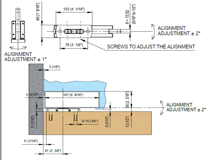
Uitsparing onderzijde 101E10 - Encoche en bas 101E10 Notch at the bottom 101E10
