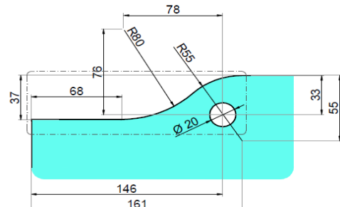
Uitsparing bovenkant 90.GHD.120D Encoche en haut 90.GHD.120D
